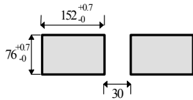
SWP - C 80.T80系列 (横式)
